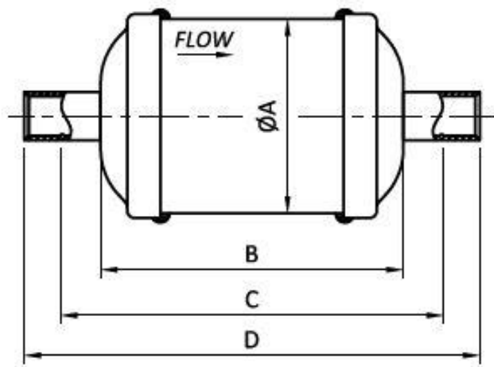
Типоразмер DFL 05-75
