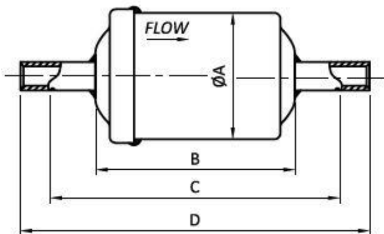
Типоразмер DFL 05-75
