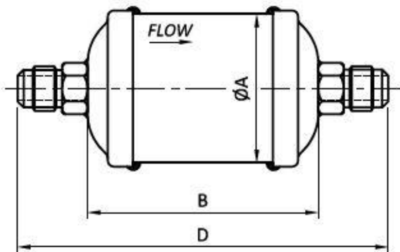
Типоразмер DGL 05-41
