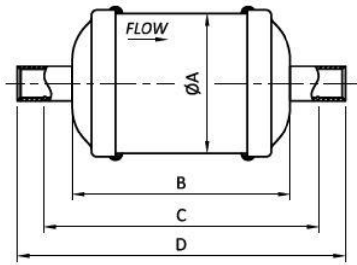
Типоразмер DFL 05-75
