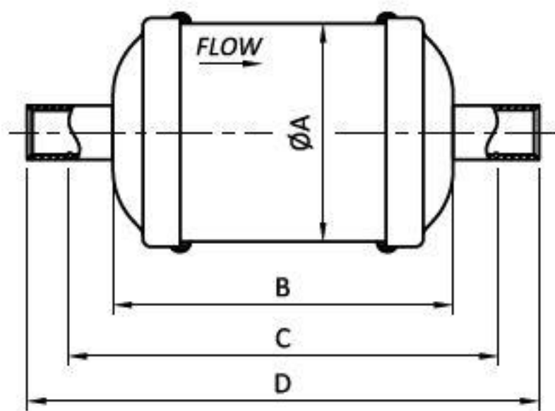
Типоразмер DGL 05-41
