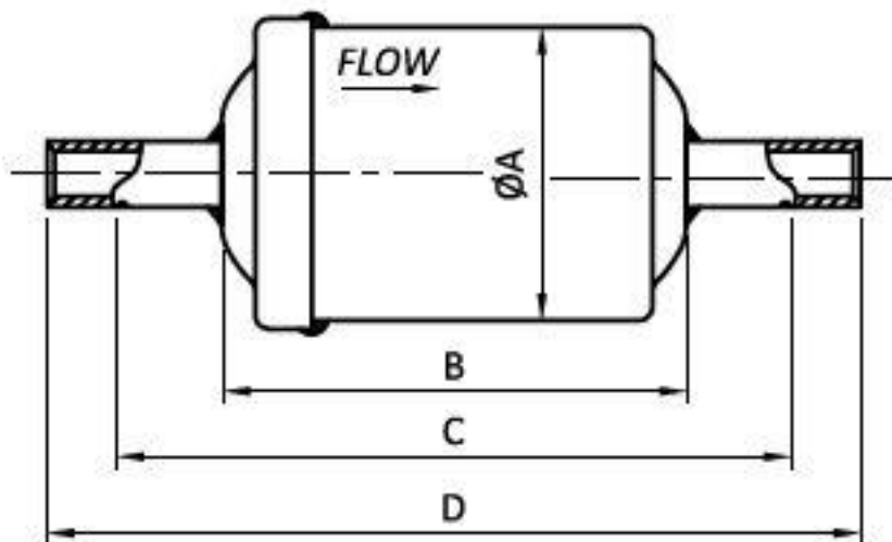
Типоразмер DGL 05-41
