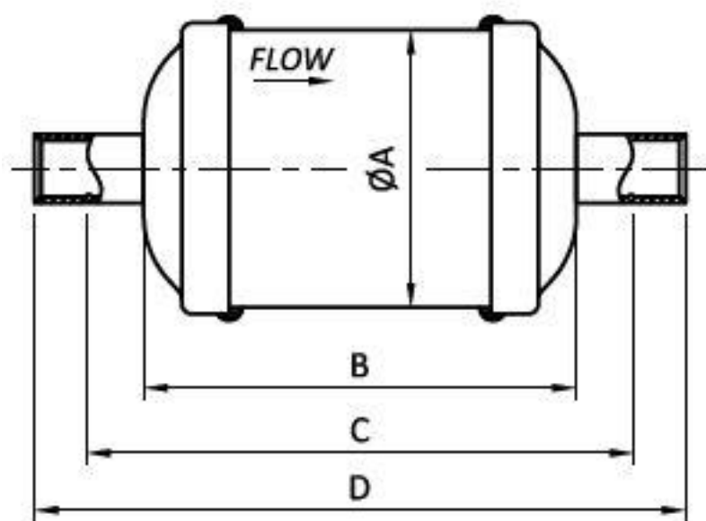
Типоразмер DGL 05-41
