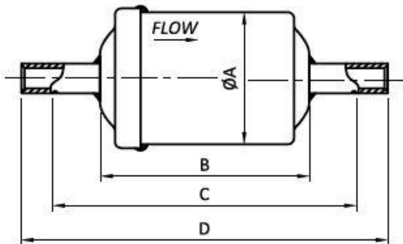
Типоразмер DGL 05-41
